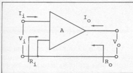
Figura 4 — Amplificador e suas variáveis de entrada e saída
